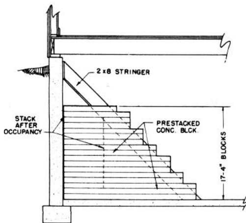
END ELEVATION
